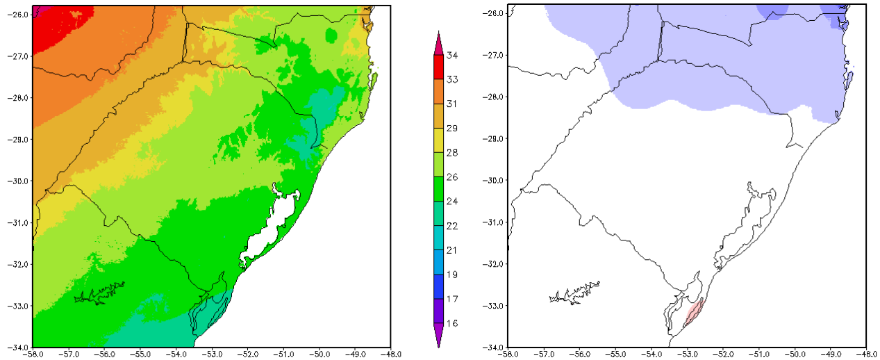
Figura 11. Temp. Máxima Média Climatologia e Anomalia Prevista Novembro/2013
