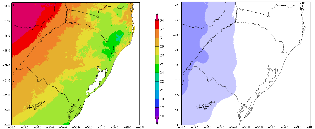
Figura 12. Temp. Máxima Média Climatologia e Anomalia Prevista Dezembro/2013
