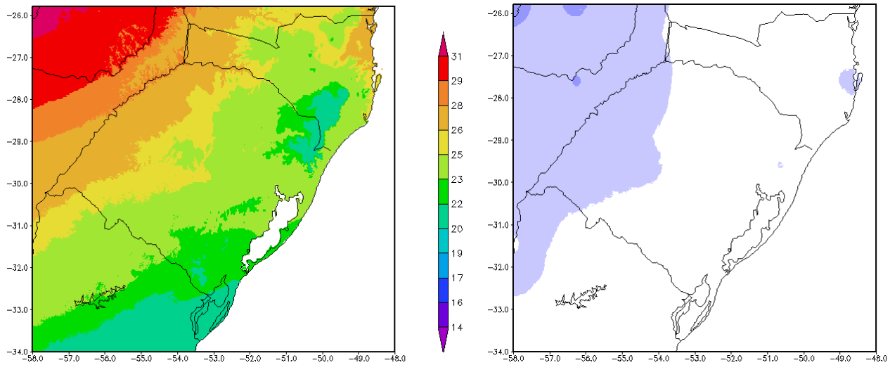
Figura 12. Temp. Máxima Média Climatologia e Anomalia Prevista Outubro/2012
